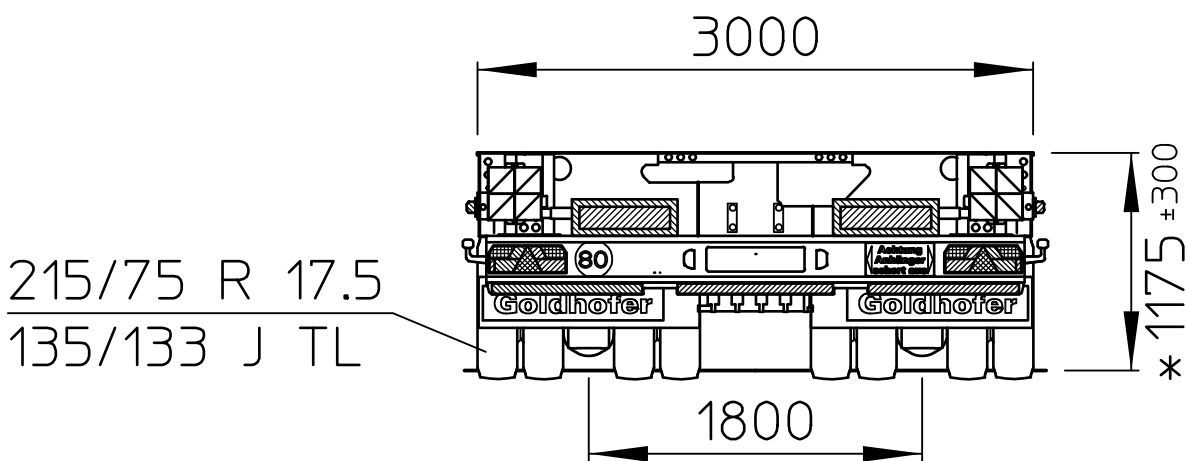
Fahrwerk Heckansicht mit Schlussstraverse
