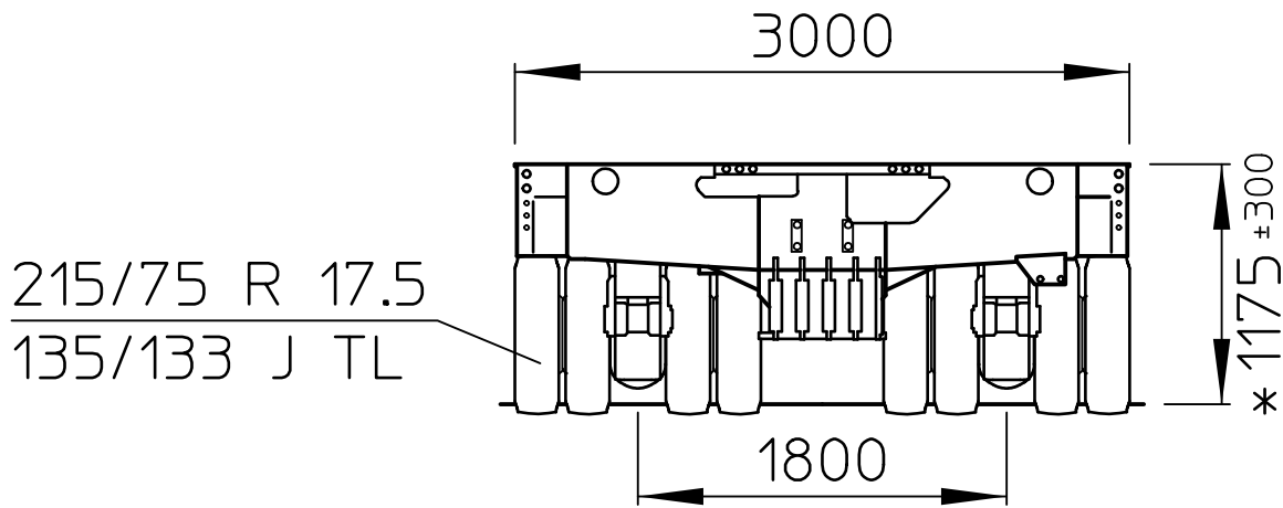
Fahrwerk Heckansicht
