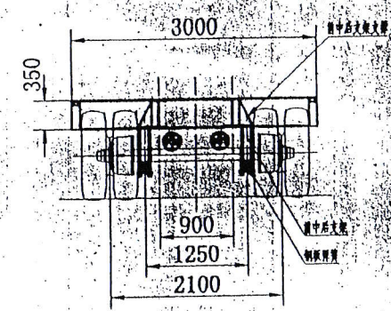
车轴段剖面
